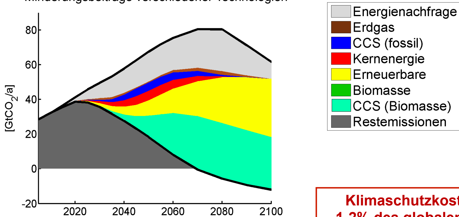
Energiebedingte CO 2 -Emissionen und Minderungsbeiträge verschiedener Technologien
